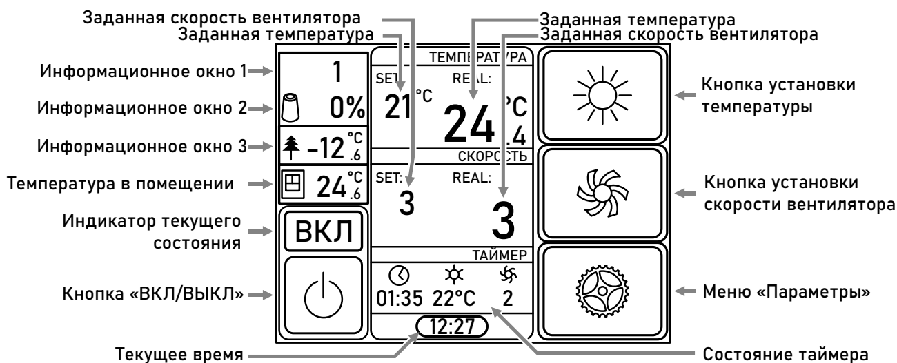
Рисунок 4 - Экран основного меню
