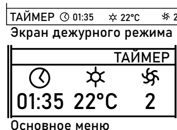
Рисунок 11 - Таймер активен, ближайшее событие на сегодня
