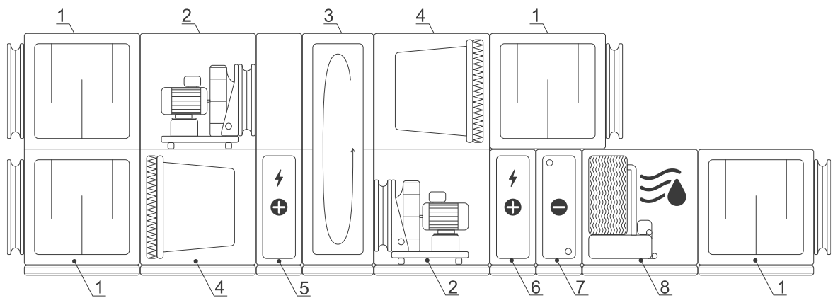
Рисунок 1 - Функциональная схема KLASIK R
