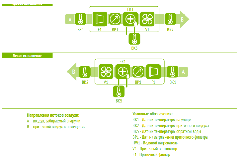
Рисунок 3. Функциональная схема установок ОТД-S-W
