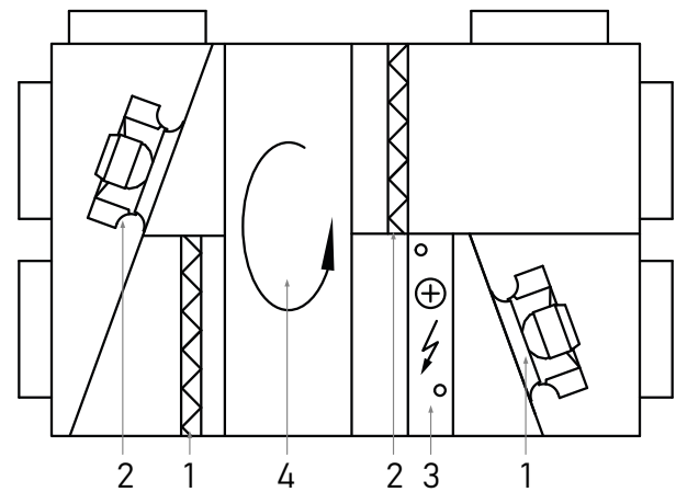
Рисунок 2 - Функциональная схема установок ОТД - R - 1000-3000 - U
