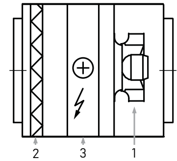
Рисунок 3 - Функциональная схема установок ОТД - S - 500-5000 - F
