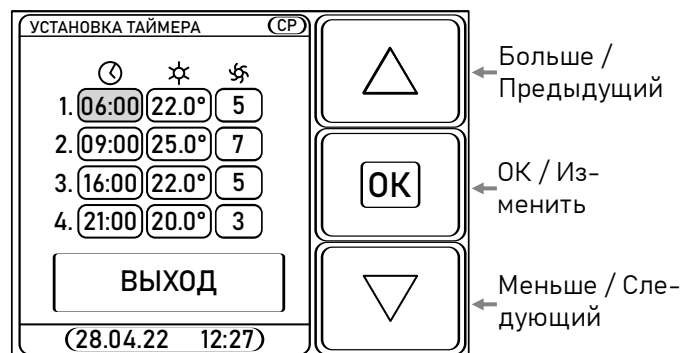
Рисунок 14 - Экран подменю установки таймеров
