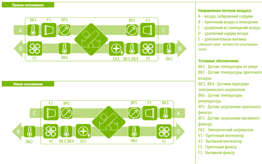
Рисунок 1. Функциональная схема установок ОТД – P-600-F
