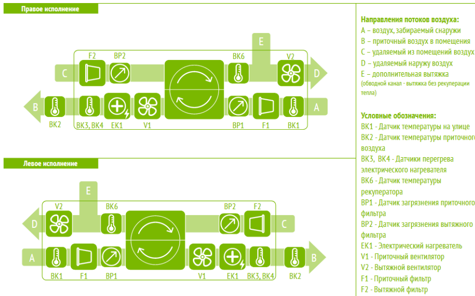
Рисунок 10. Функциональная схема установок ОТД-R-250-F
