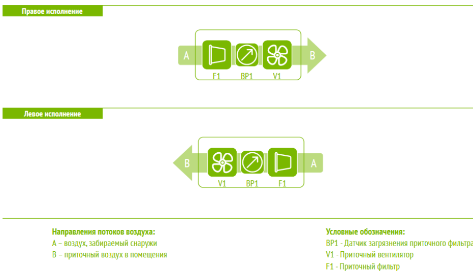
Рисунок 12. Функциональная схема установок ОТД-S-X
