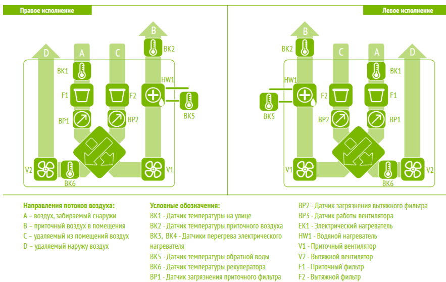
Рисунок 2. Функциональная схема установок ОТД – P-...-V-W
