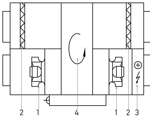
Рисунок 1 - Функциональная схема установок ОТД - R - 400-1300 - F
